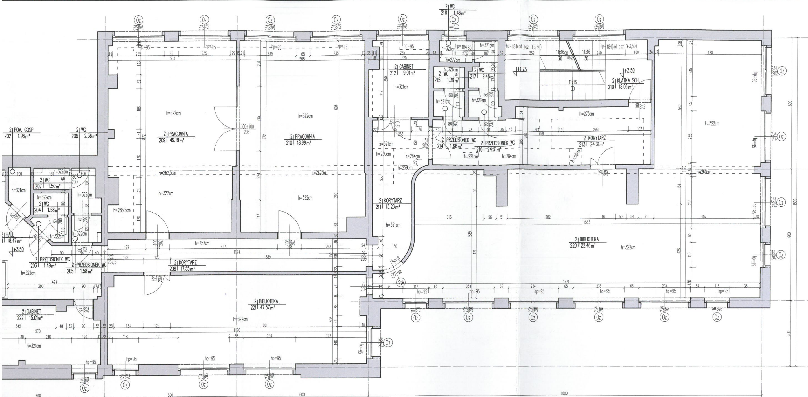
RZUT KONDYGNACJI 2 SKALA 1:100
